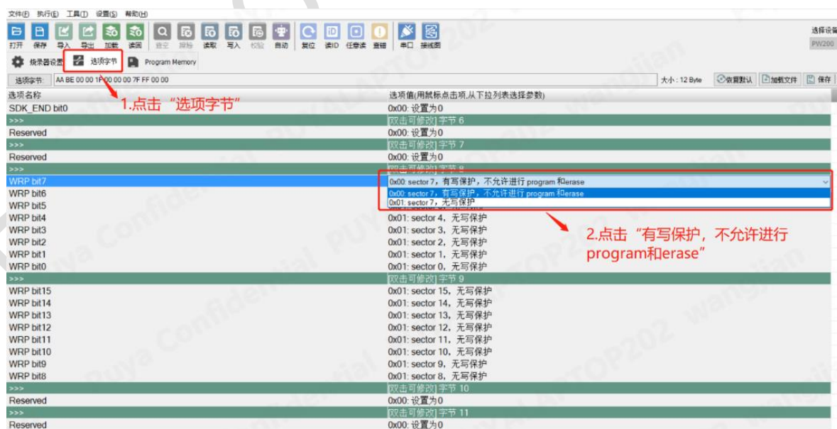
图 17-2 创芯工坊操作 Option 写保护
